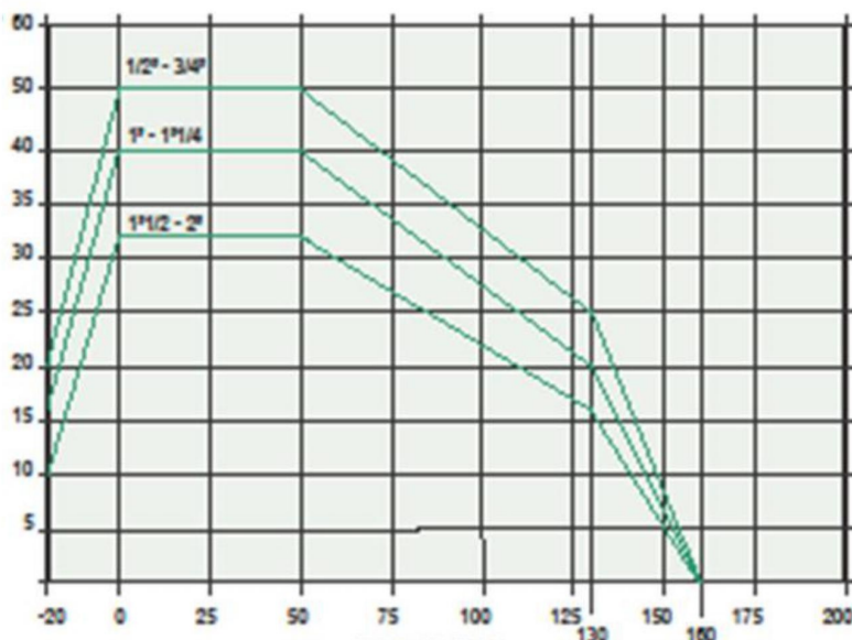
Рис.1.1. Зависимость рабочего давления от температуры перемещаемой среды
