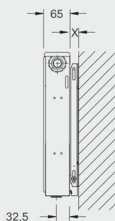
Вид сбоку Тип 10
