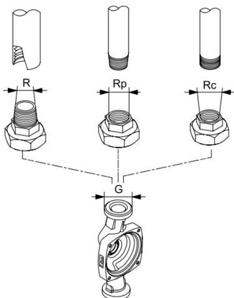
Рис. 18 Резьба G и резьба R
