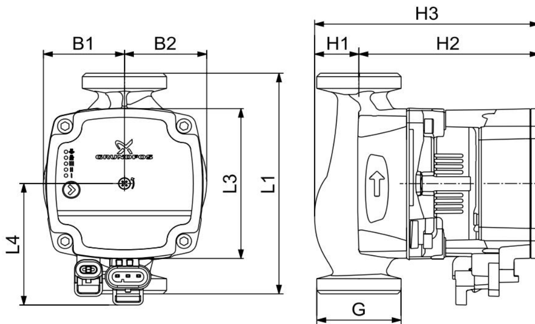
Рис. 16 Габаритные размеры
