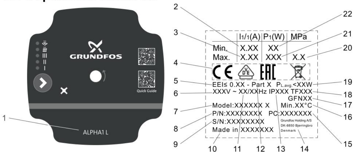
Рис. 1 Фирменная табличка насоса ALPHA1 L
