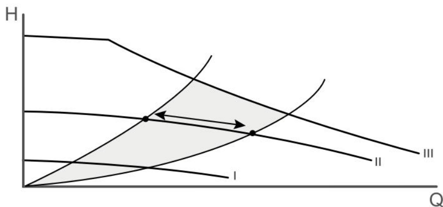
Рис. 13 Пример трёх кривых фиксированных скоростей
