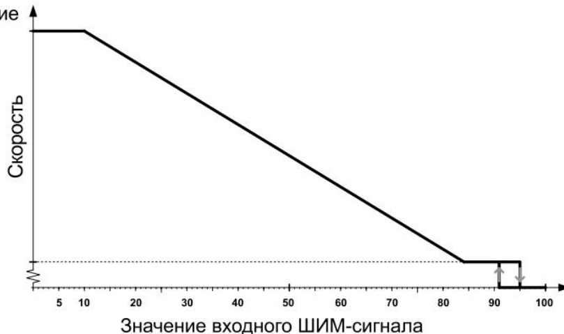
Рис. 14 Профиль ШИМ-сигнала
