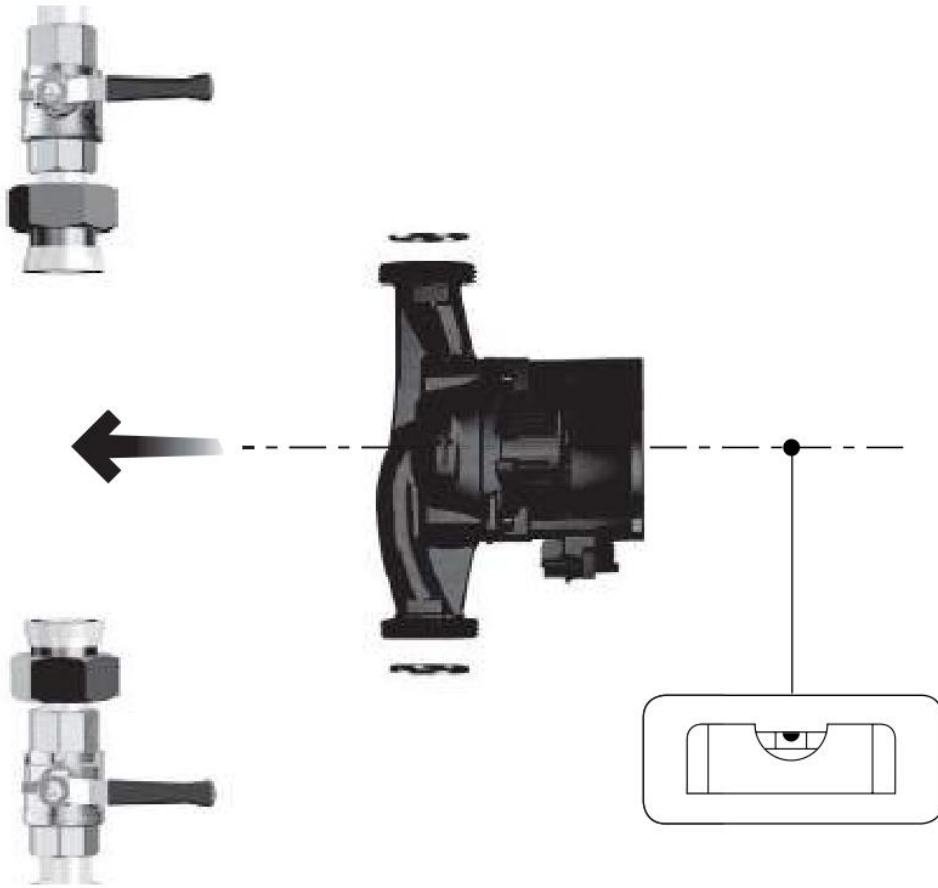
Рис. 3 Монтаж насоса
