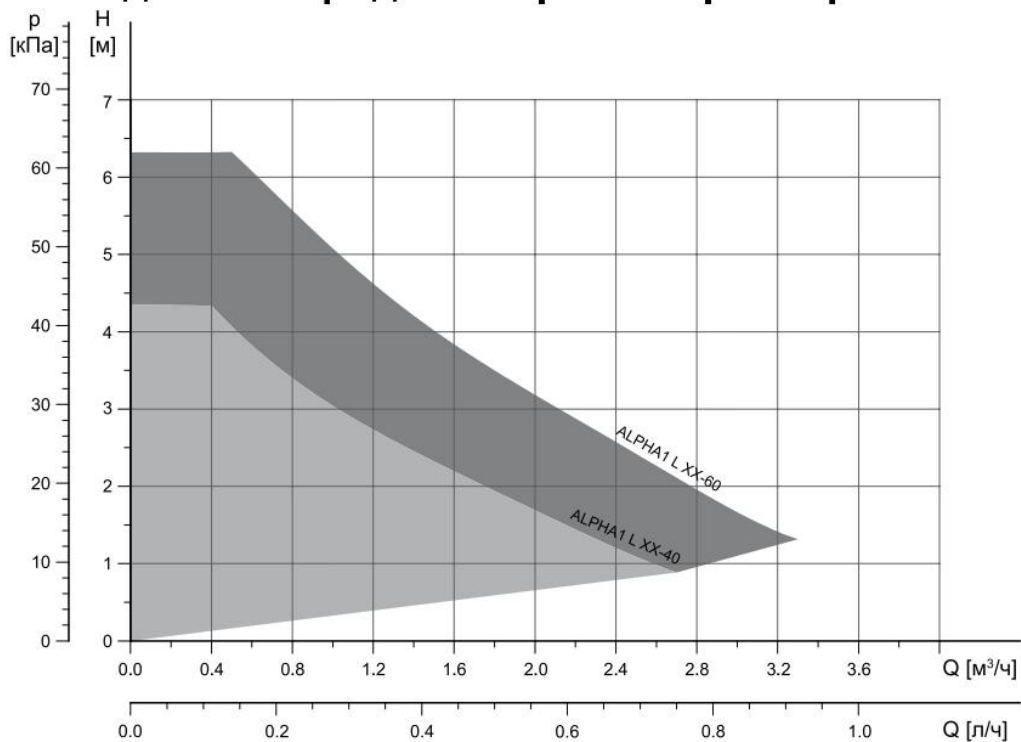
Рис. 15 Расходно-напорная характеристика насосов серии ALPHA1 L
