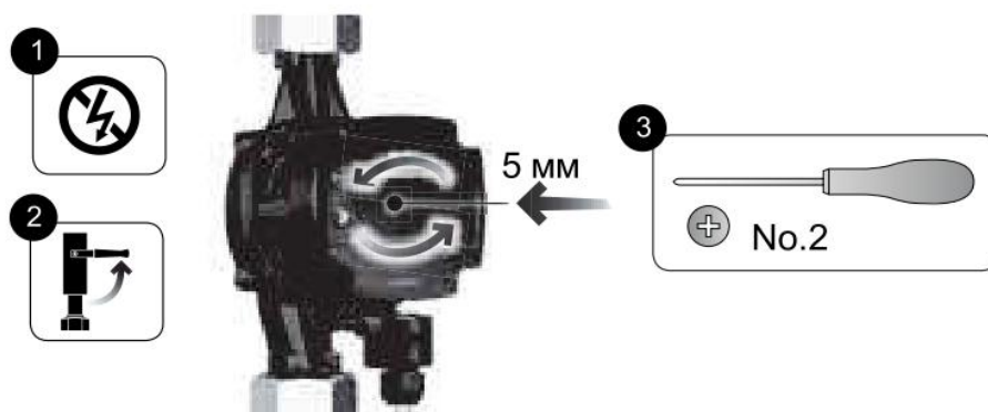
Рис. 17 Разблокировка вала
