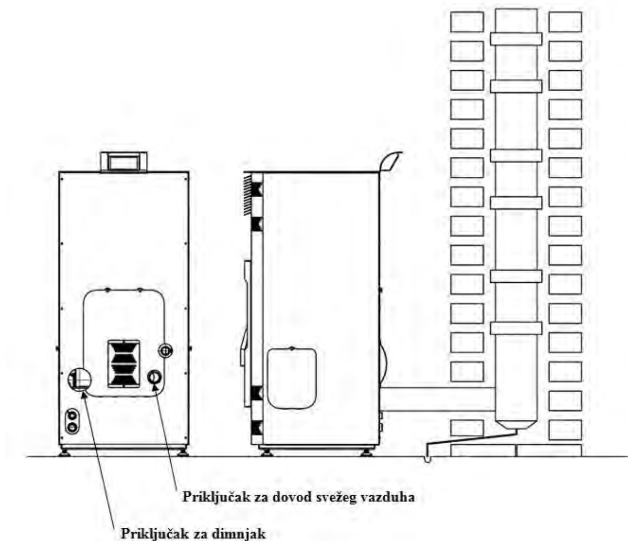
Рис 8. Вид подключения к дымоходу и отображения положения зонда в дымоходе
