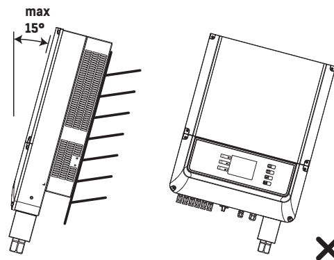
Рисунок 3.4.2 Установка инвертора на поверхность
