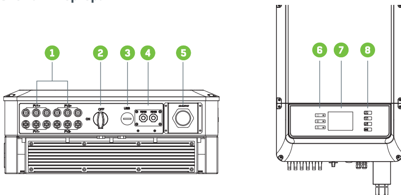
Рисунок 2.3.1 Схема инвертора
