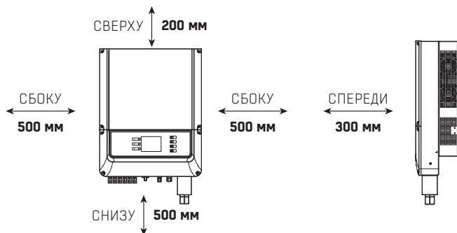
Рисунок 3.4.3 Расстояния до места установки инвертора
