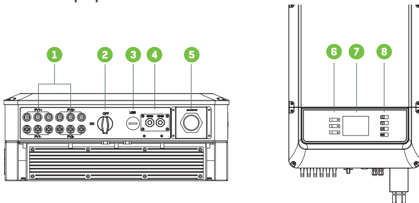
Рисунок 2.3.1 Схема инвертора
