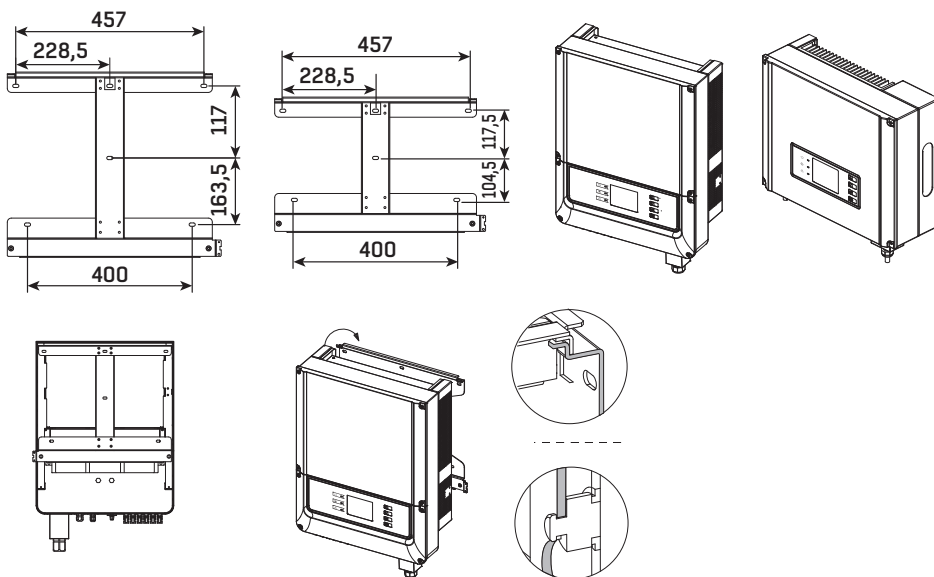
Рисунок 3.4.4 Инструкция по креплению инвертора на поверхность
